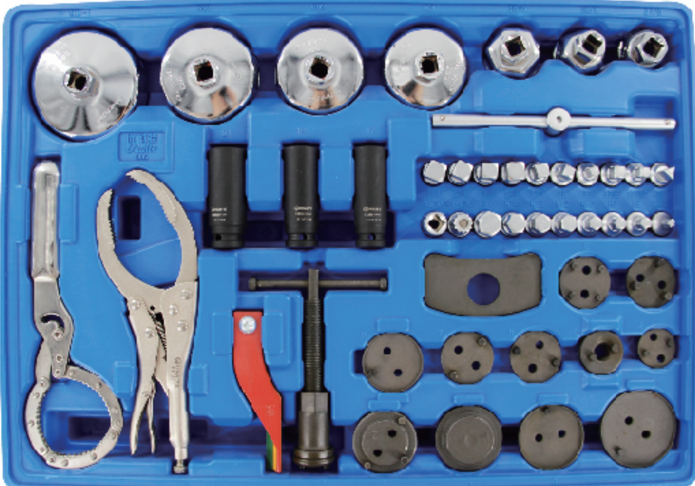
170803 47件快保工具
